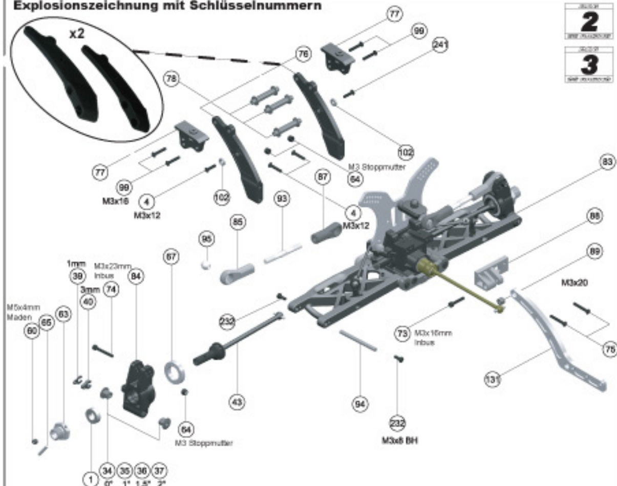
Explosionszeichnung mit Schlüsselnummern
